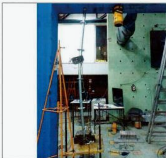
Fotografía 7.2.2.1: Probeta CPD-RD66-01 durante el ensayo
